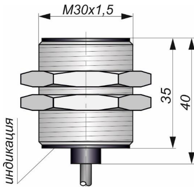
Габаритный чертеж
